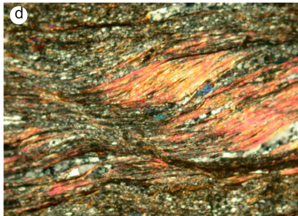
Fig.8 - Microstrutture prodotte dall'evento deformativo di taglio duttile nei litotipi paraderivati: (a-b) strutture e paragenesi relitte in low strain domain all'interno degli orizzonti metapelitici; (c) biotiti con tessiture tipo fish definenti un senso di taglio destro; (d) foliation fish rappresentate da lenti policristalline di mica chiara in metapelite; (e) porfiroclasto sigmoide di plagioclasio in metapelite.
