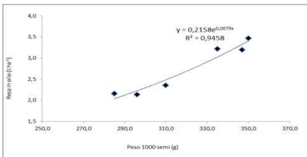
Fig. 10.25 Correlazione tra peso 1000 semi e resa in olio nell'anno 2008 ( r = 0,968837 ; p = 0,0003 ).
