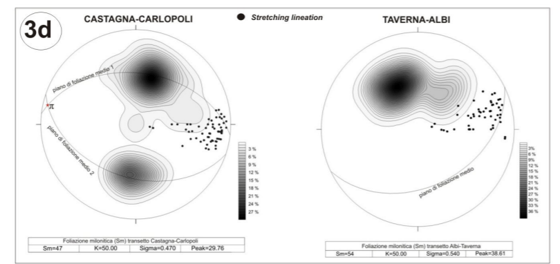
Distribuzione dei poli dei piani relativi alla foliazione milonitica nei litotipi gneissici dell'Unità di Castagna relativamente alle due aree indagate. Equal-area projection plots(Lower hemisphere)
