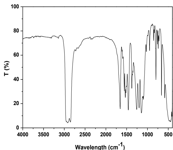
Fig. 2.3.1.3 FT-IR spectrum of complex [Y(hfa)_4]^- [Na \cdot tetraglyme]^+
