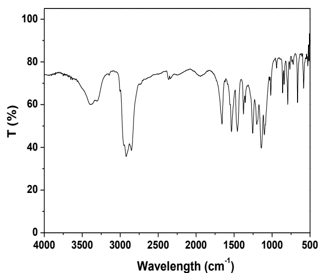
Fig 2.1.2.1 FT-IR spectrum of Mg(hfa) 2 ·2H 2 O·2diglyme.
