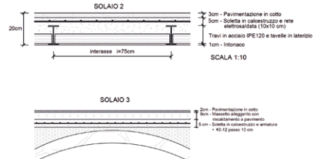
Dettaglio orizzontamenti
