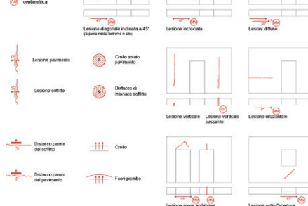
3. Rilievo materico-costruttivo e quadro fessurativo
