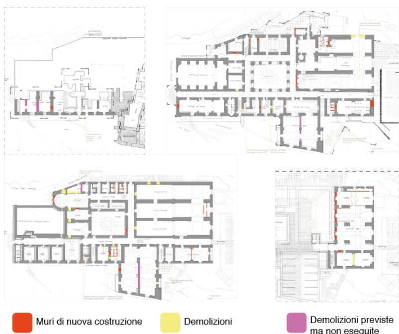
Figura 4.16 - Studio preliminare rilievi. La sovrapposizione delle planimetrie attuali e quelle del progetto di restauro degli anni '80 mette in evidenza alcune trasformazioni (demolizioni di muri, nuovi varchi, ecc.) attuate nel palazzo per la nuova destinazione d'uso museale.
