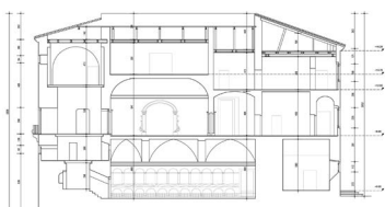
sezione 1_1
