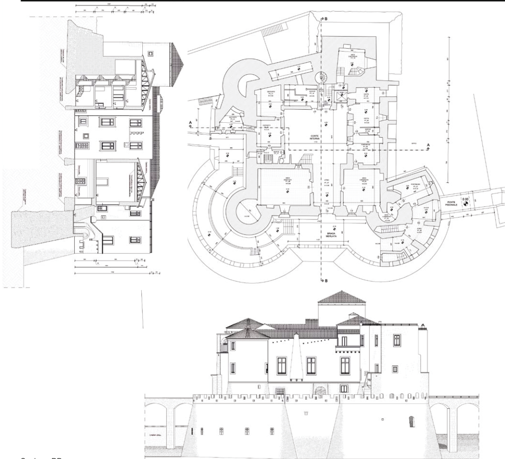
Sezione BB
