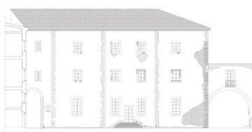
prospetto sud
