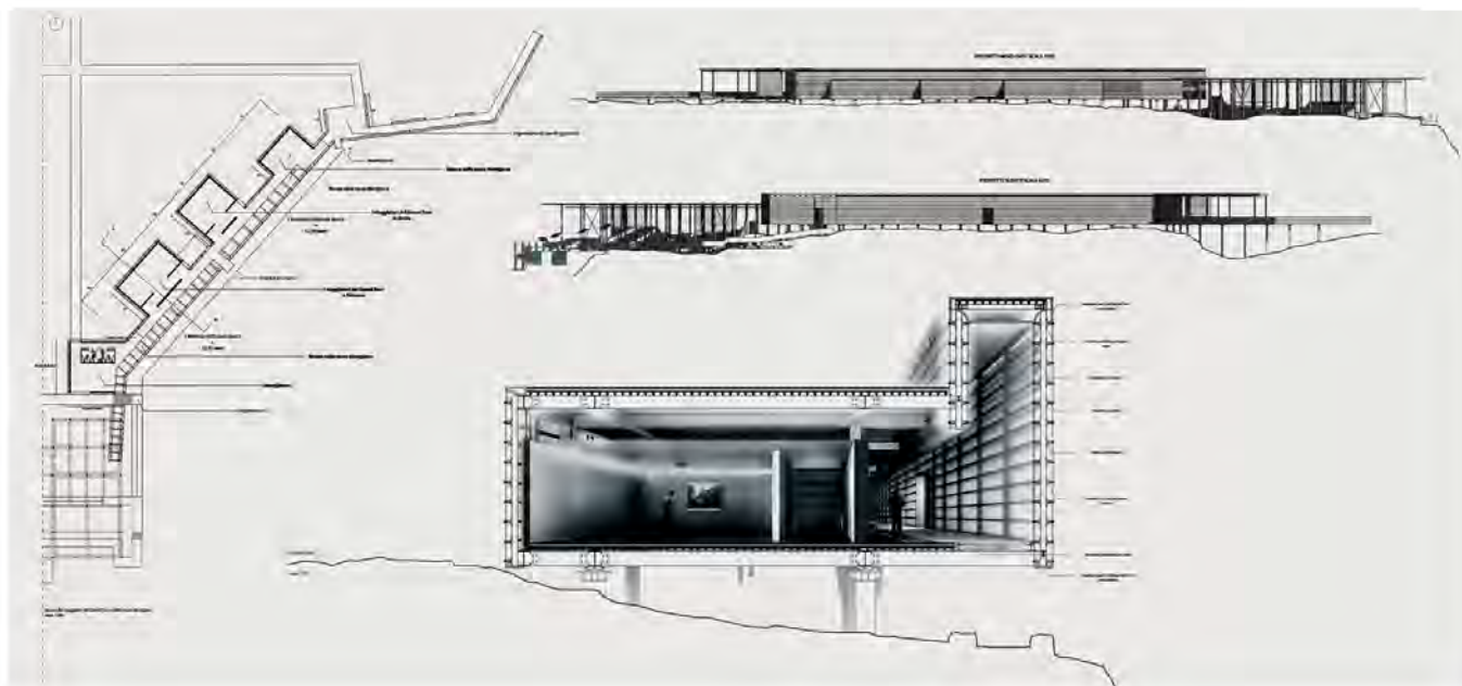
[16] MASSIMILIANO OSSINO, SDS SIRACUSA, TESI DI LAUREA A.A. 2014-2015, MUSEO, PIANTA, PROSPETTO E SEZIONE PROSPETTICA.
