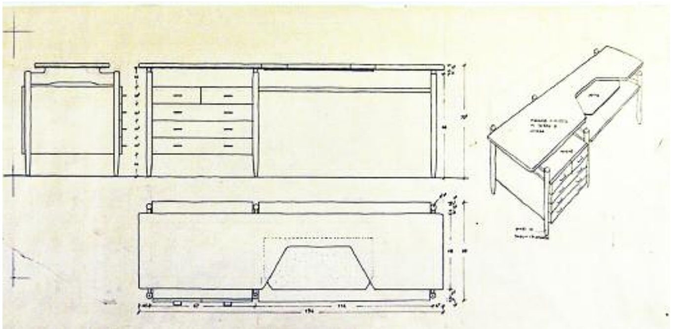
82/ Dettaglio del modile da toilette della casa Caruso a Valdesi Mondello , G. Pirrone, 1957 (n. inv. 16-PRA-21).
