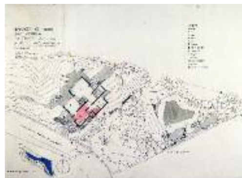
112/ Planimetria della casa sul mare ad Altavilla Milicia, G. Pirrone con G. Ferla, 1967-71 (n. inv. 29-P-02a).
