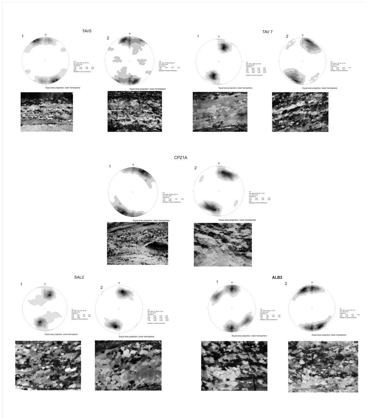
Fig.7 Microdomini di quarzo in campioni di para ed ortoderivati dell'Unità di Castagna con relativi patterns coerenti con un single girdle di bassa temperatura indicativi di condizioni tipiche della green schist facies inferiore (400-450°).
