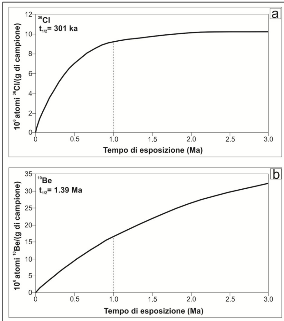
Fig. 75- Influenza del tempo di dimezzamento sul tempo di esposizione e sul raggiungimento dello steady state.
