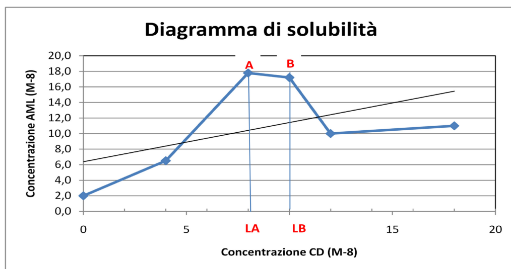
Figura 22: Diagramma di solubilità
