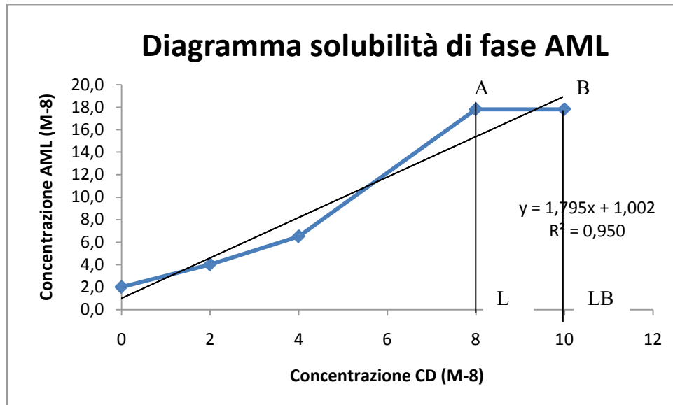
Figura 23: Diagramma solubilità di fase AML
