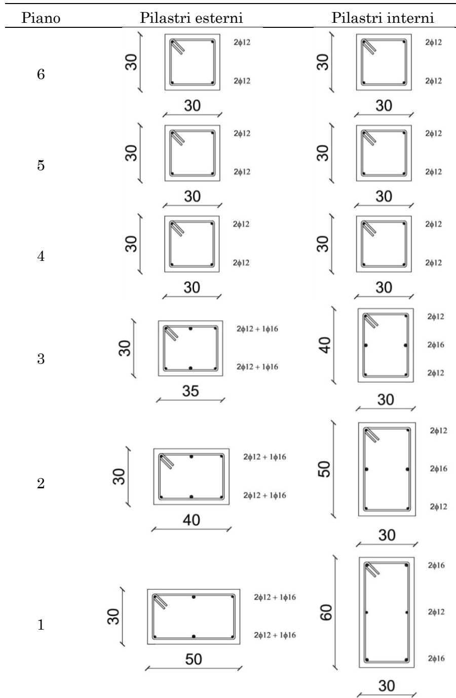
Figura 35 – Sezioni dei pilastri per il telaio progettato per c.v.
