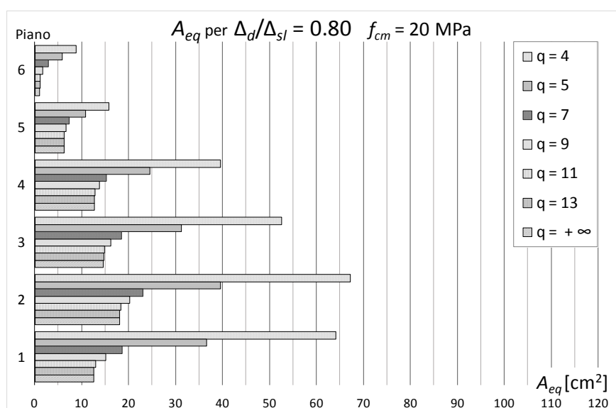
Figura 109 – Aree equivalenti per progetti sul telaio CV2 ( f_{cm} = 20 MPa) con (\Delta_d / \Delta_{SL})_i = 0.8 al variare di q
