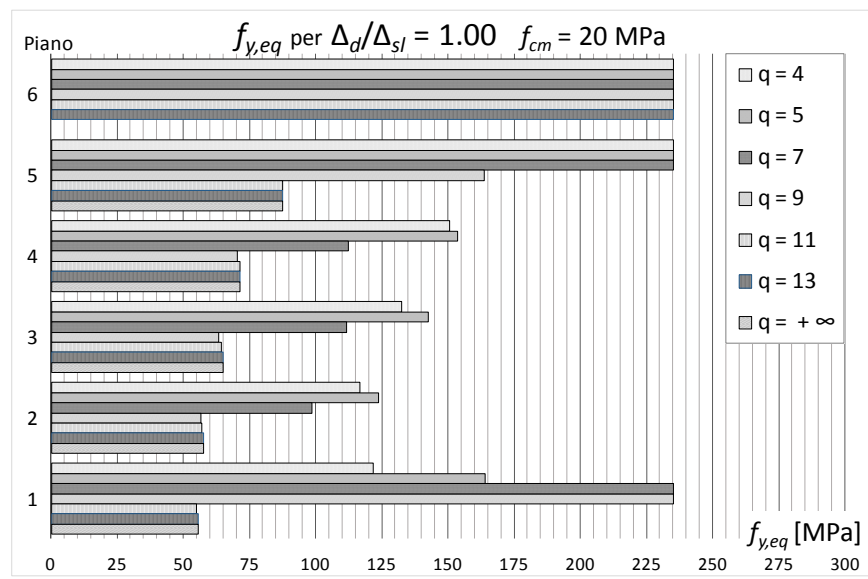
Figura 113 – Tensioni di snervamento equivalenti per progetti sul telaio CV2 ( f_{cm} = 20 MPa) con (\Delta_d/\Delta_{sl})_i = 1.0 al variare di q
