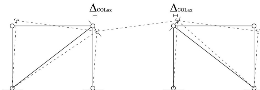
Figura 15 – Drift dovuti alla deformabilità assiale dei pilastri
