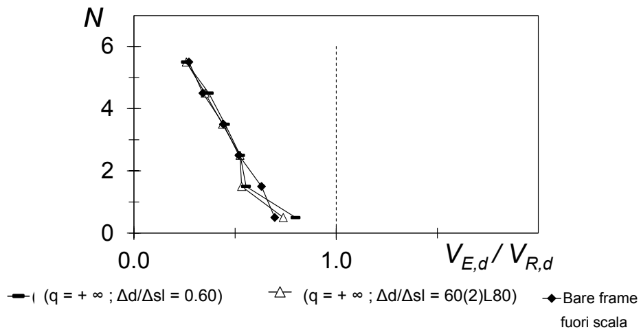
Figura 87 – Massimo rapporto V_{Ed} / V_{Rd} fra taglio sollecitante e resistente per il telaio CV2 con f_{cm} = 20 MPa adeguato, con distribuzione del rapporto (\Delta d/\Delta sL)_i costante e pari a 0.60 oppure di tipo 60(2)L80
