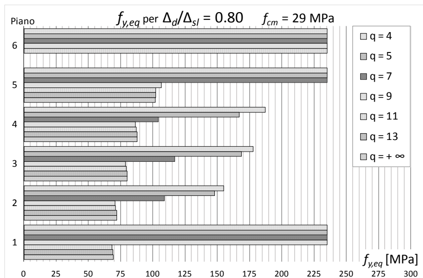
Figura 103 – Tensioni di snervamento equivalenti per progetti sul telaio CV1 ( f_{cm} = 29 MPa) con (\Delta_d/\Delta_{SL})_i = 0.8 al variare di q
