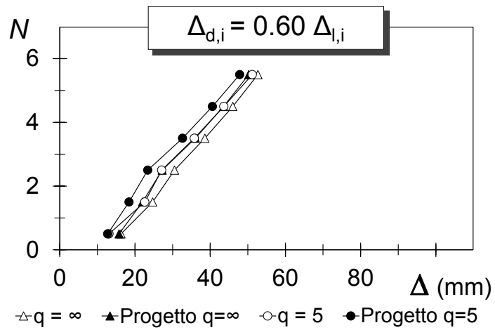
Figura 94 – Capacità di spostamento di interpiano \Delta_{SL} : confronto fra previsione in fase progettuale e capacità ottenuta con ADNL per il telaio AS con f_{cm} = 20 MPa adeguato, con (\Delta_d/\Delta_{SL})_i = 0.60
