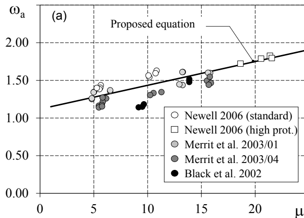
Figura 11 – Fattore \omega_a per la modellazione del comportamento inelastico dei BRBs 14,15
