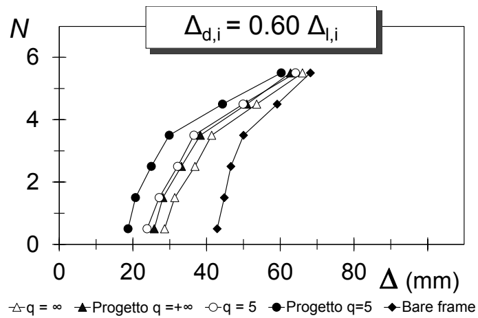
Figura 78 – Capacità di spostamento di interpiano \Delta_{SL} : confronto fra previsione in fase progettuale e capacità ottenuta con ADNL per il telaio CV2 con f_{cm} = 20 MPa adeguato, con (\Delta_d/\Delta_{SL})_i = 0.60
