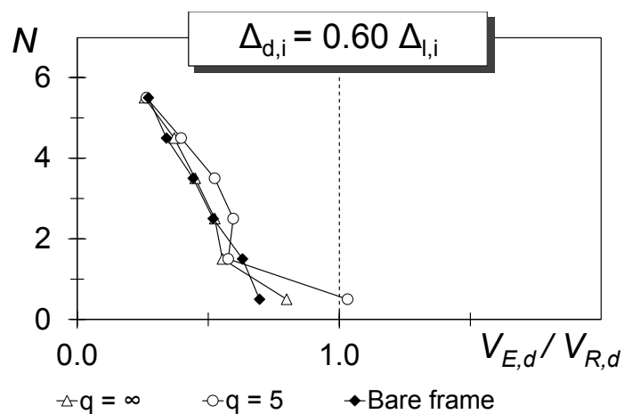
Figura 80 – Massimo rapporto V_{Ed}/V_{Rd} fra taglio sollecitante e resistente per il telaio CV2 con f_{cm} = 20 MPa adeguato, con (\Delta_d/\Delta_{sl})_i = 0.60
