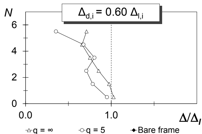
Figura 75 – Massimo rapporto \Delta/\Delta_{SL} per il telaio CV2 con f_{cm} = 20 MPa adeguato, con (\Delta_d/\Delta_{SL})_i = 0.60
