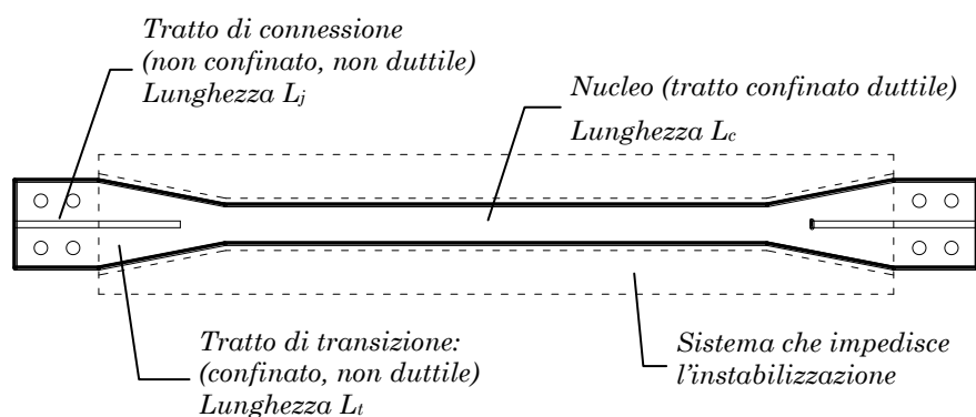
Figura 5 – Componenti di un controvento a instabilità impedita
