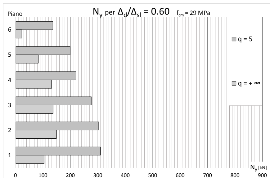
Figura 65 – Resistenze allo snervamento N_y dei BRBs per il telaio CV1 con f_{cm} = 29 MPa adeguato, con (\Delta_d/\Delta_{sl})_i = 0.60
