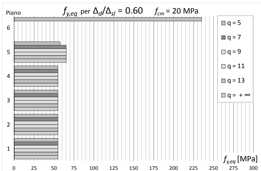
Figura 118 – Tensioni di snervamento equivalenti per progetti sul telaio AS ( f_{cm} = 20 MPa) con (\Delta_d/\Delta_{SL})_i = 0.6 al variare di q
