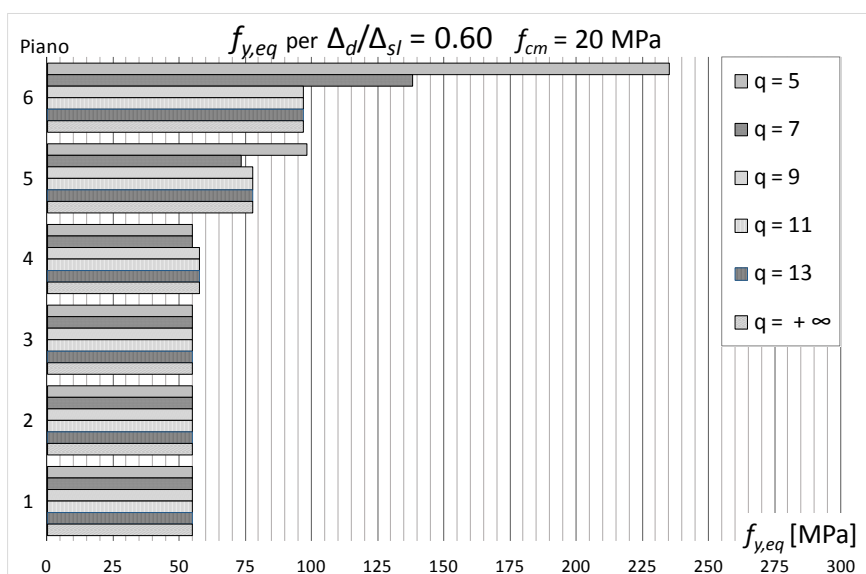
Figura 111 – Tensioni di snervamento equivalenti per progetti sul telaio CV2 ( f_{cm} = 20 MPa) con (\Delta_d / \Delta_{SL})_i = 0.6 al variare di q
