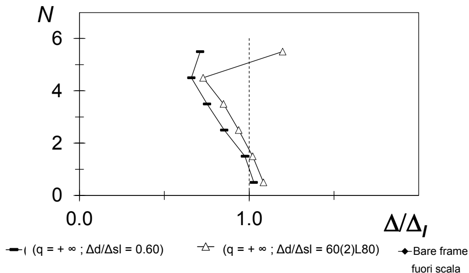
Figura 83 – Massimo rapporto \Delta/\Delta_{SL} per il telaio CV2 con f_{cm} = 20 MPa adeguato, con distribuzione del rapporto ( \Delta_d/\Delta_{SL} );
