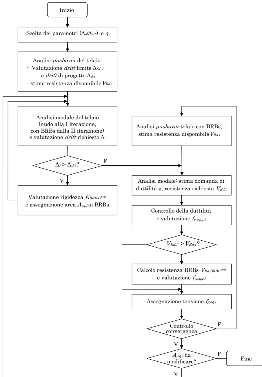
Figura 19 – Diagramma di flusso del metodo di progetto
