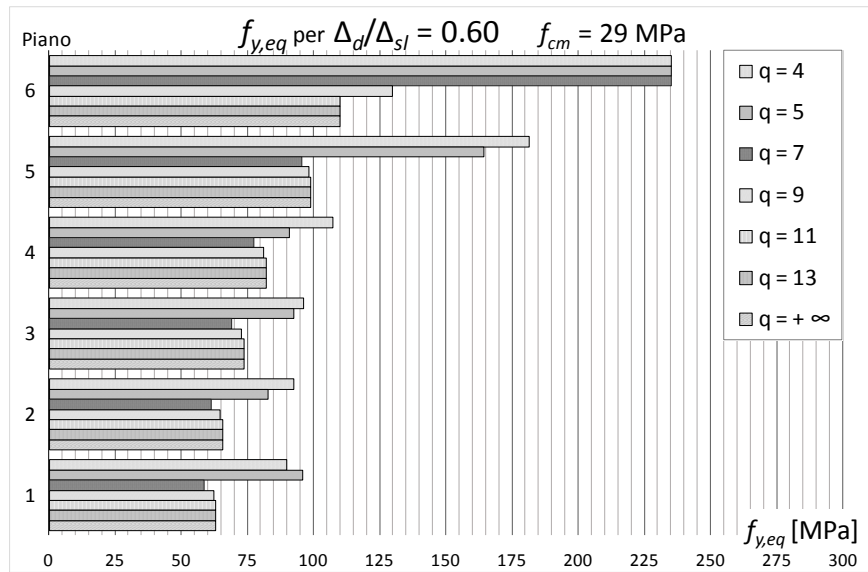
Figura 102 – Tensioni di snervamento equivalenti per progetti sul telaio CV1 ( f_{cm} = 29 MPa) con (\Delta_d/\Delta_{SL})_i = 0.6 al variare di q
