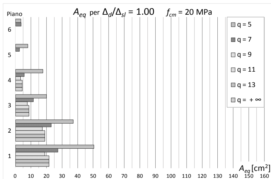
Figura 117 – Aree equivalenti per progetti sul telaio AS ( f_{cm} = 20 \text{ MPa} ) con (\Delta_d / \Delta_{SL})_i = 1.0 al variare di q
