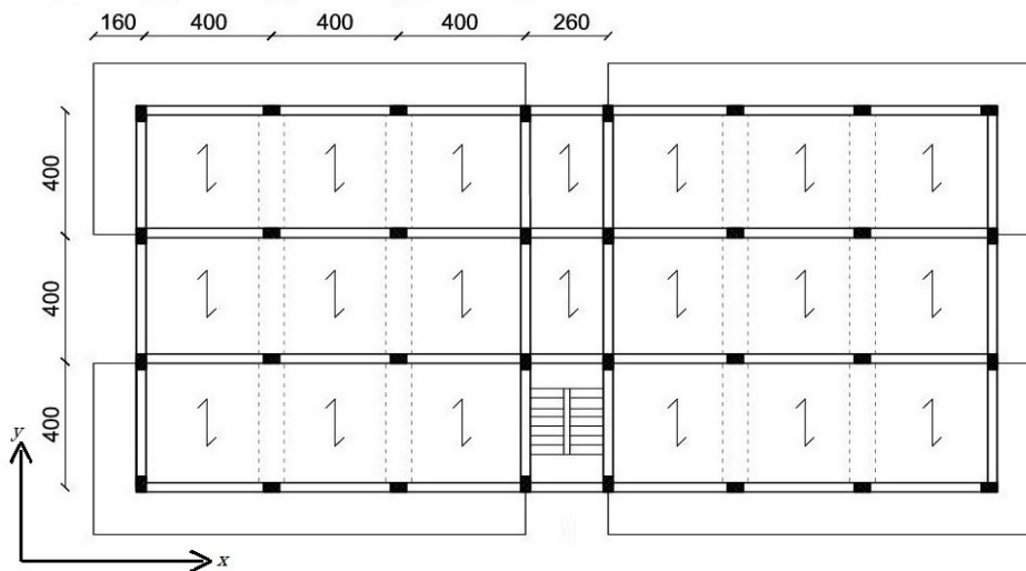
Figura 36 – Pianta dell'edificio progettato per zone a bassa sismicità
