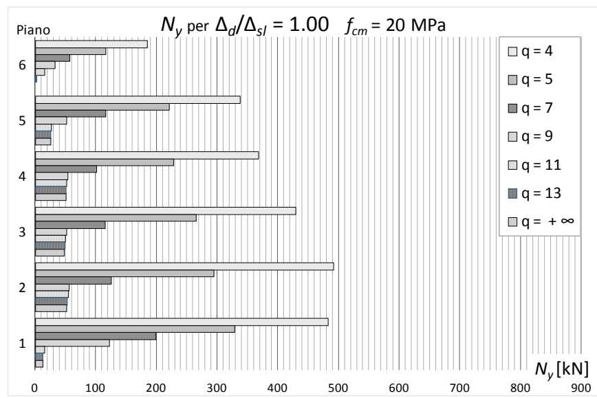
Figura 116 – Resistenza allo snervamento per progetti sul telaio CV2 ( f_{cm} = 20 MPa) con (\Delta_d/\Delta_{SL})_i = 1.0 al variare di q
