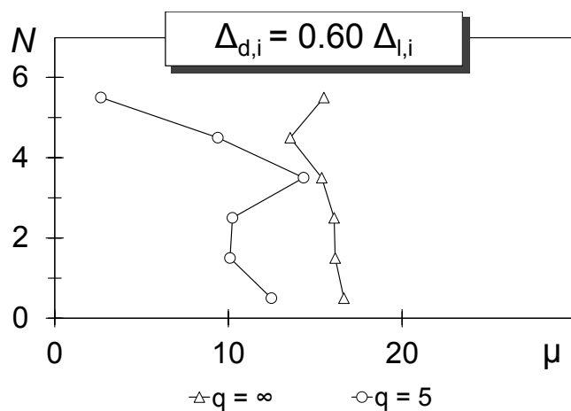
Figura 79 – Massima duttilità \mu richiesta ai BRBs per il telaio CV2 con f_{cm} = 20 MPa adeguato, con (\Delta_d/\Delta_{sl})_i = 0.60
