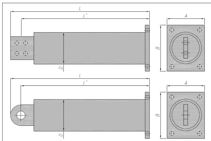
Figura 8 – Schema geometrico dei controventi BRAD® prodotti da FIP industriale
