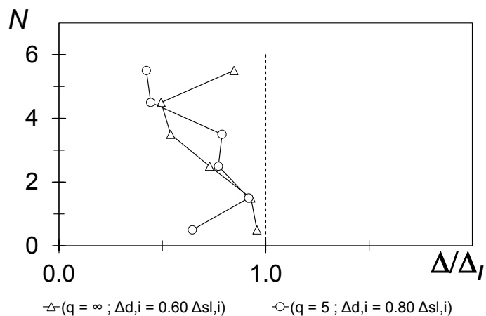
Figura 66 – Massimo rapporto \Delta/\Delta_{SL} per il telaio CV1 con f_{cm} = 29 MPa adeguato, con (\Delta_d / \Delta_{SL})_i = 0.6 , q = +\infty oppure (\Delta_d / \Delta_{SL})_i = 0.8 , q = 5
