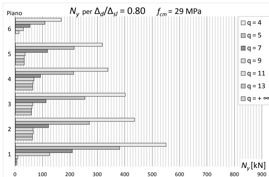
Figura 106 – Resistenza allo snervamento per progetti sul telaio CV1 ( f_{cm} = 29 MPa) con (\Delta_d/\Delta_{SL})_i = 0.8 al variare di q
