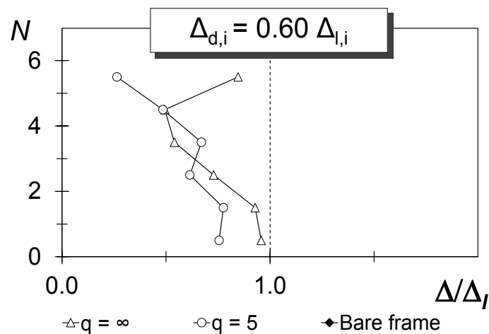
Figura 58 – Massimo rapporto \Delta/\Delta_{SL} per il telaio CV1 con f_{cm} = 29 MPa adeguato, con (\Delta_d/\Delta_{SL})_i = 0.60
