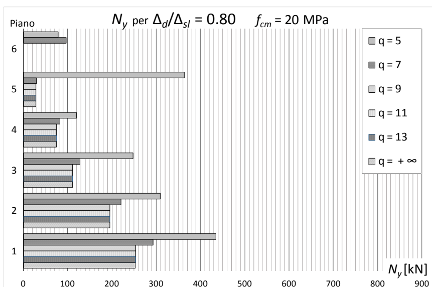
Figura 121 – Resistenza allo snervamento per progetti sul telaio AS ( f_{cm} = 20 MPa) con (\Delta_d / \Delta_{SL})_i = 0.8 al variare di q
