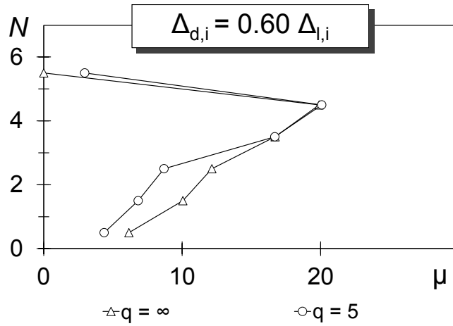
Figura 95 – Massima duttilità \mu richiesta ai BRBs per il telaio CV1 con f_{cm} = 29 MPa adeguato, con (\Delta_d/\Delta_{SL})_i = 0.60
