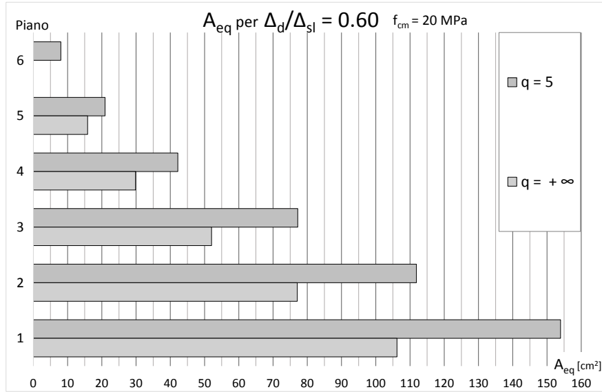
Figura 97 – Aree equivalenti A_{eq} dei BRBs per il telaio AS con f_{cm} = 20 MPa adeguato, con (\Delta_d/\Delta_{SL})_i = 0.6
