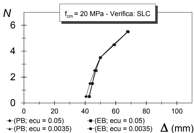
Figura 74 – Capacità di spostamento di interpiano \Delta_{SL} in corrispondenza del massimo rapporto domanda/capacità di spostamento per il telaio CV2
