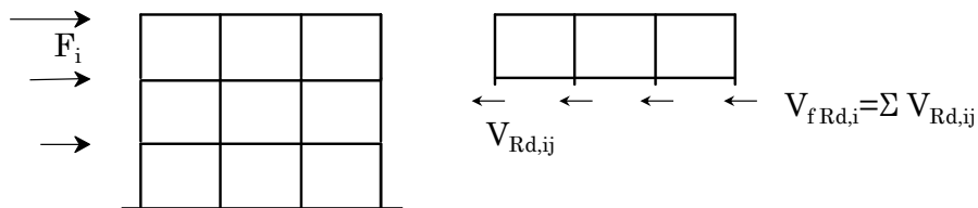
Figura 17 – Resistenza a taglio del telaio nudo in c.a.
