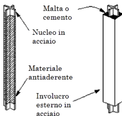
Figura 4 – Controventi a instabilità impedita
