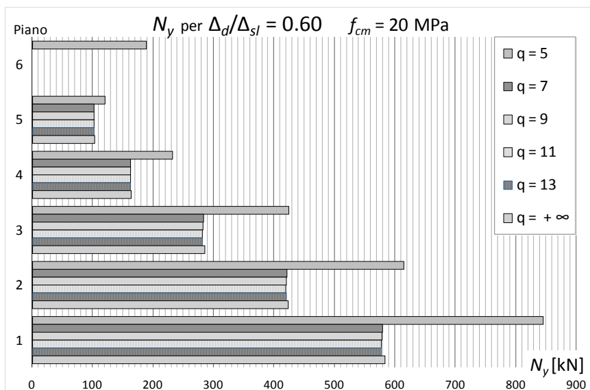
Figura 120 – Resistenza allo snervamento per progetti sul telaio AS ( f_{cm} = 20 MPa) con (\Delta_d / \Delta_{SL})_i = 0.6 al variare di q
