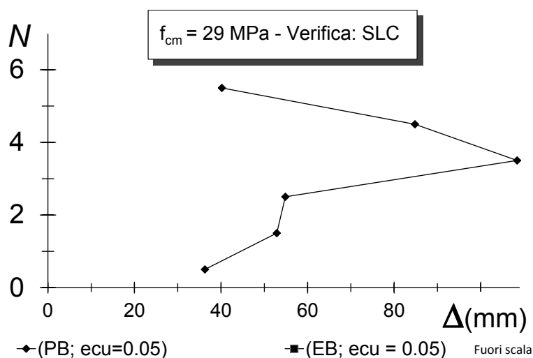
Figura 55 – Massimi spostamenti di interpiano richiesti per il telaio nudo CV1
