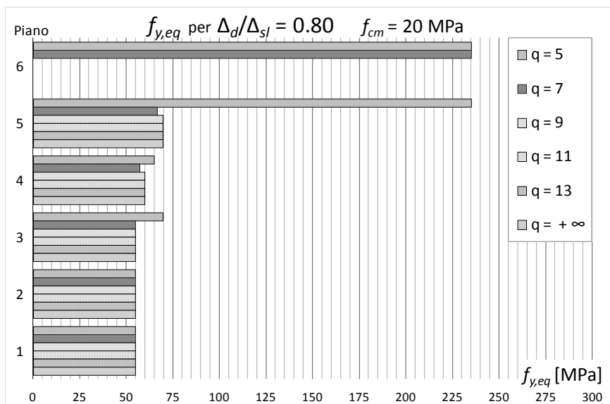
Figura 119 – Tensioni di snervamento equivalenti per progetti sul telaio AS ( f_{cm} = 20 MPa) con (\Delta_d/\Delta_{SL})_i = 0.8 al variare di q
