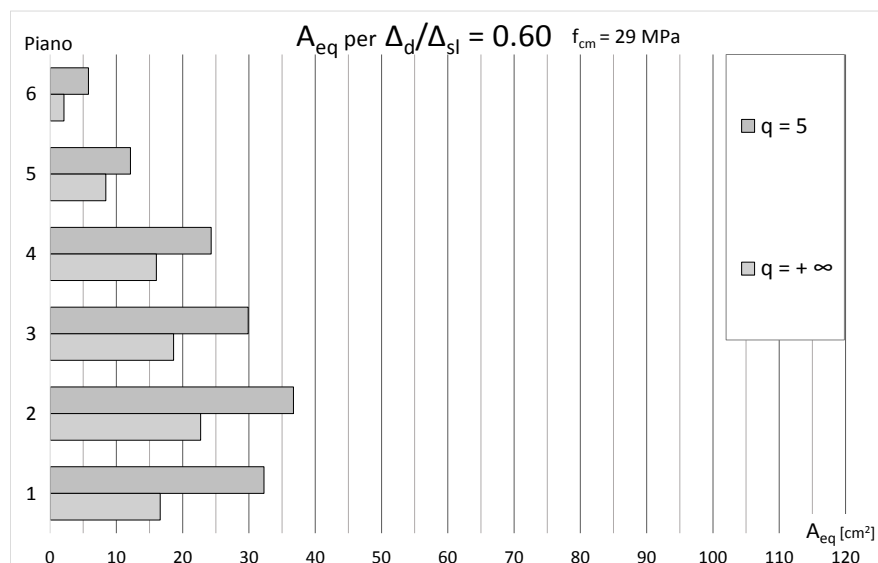
Figura 64 – Aree equivalenti A_{eq} dei BRBs per il telaio CV1 con f_{cm} = 29 MPa adeguato, con (\Delta_d/\Delta_{sl})_i = 0.60
