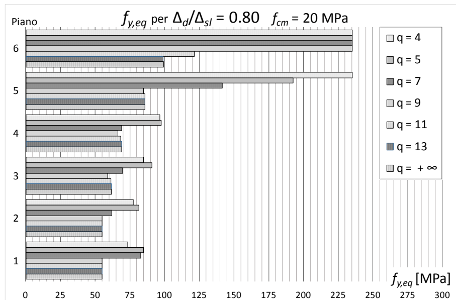
Figura 44 – Aree equivalenti per progetti sul telaio CV2 ( f_{cm} = 20 MPa) con (\Delta_d / \Delta_{SL})_i = 0.8 al variare di q
