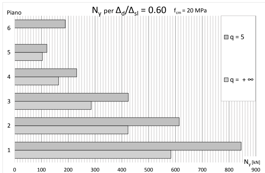
Figura 98 – Resistenze allo snervamento N_y dei BRBs per il telaio AS con f_{cm} = 20 MPa adeguato, con (\Delta_d/\Delta_{SL})_i = 0.6
