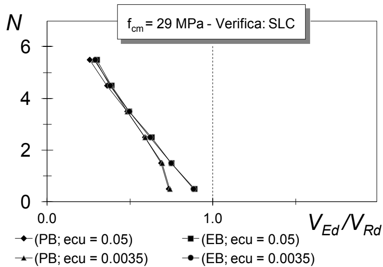
Figura 57 – Rapporto taglio sollecitante/resistente per il telaio nudo CV1
