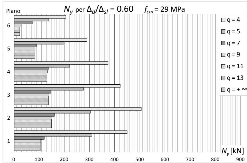
Figura 105 – Resistenza allo snervamento per progetti sul telaio CV1 ( f_{cm} = 29 MPa) con (\Delta_d/\Delta_{SL})_i = 0.6 al variare di q
