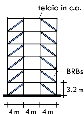
Figura 33 – Telaio estratto dall'edificio esistente: schema geometrico del telaio in c.a. con disposizione dei BRBs
