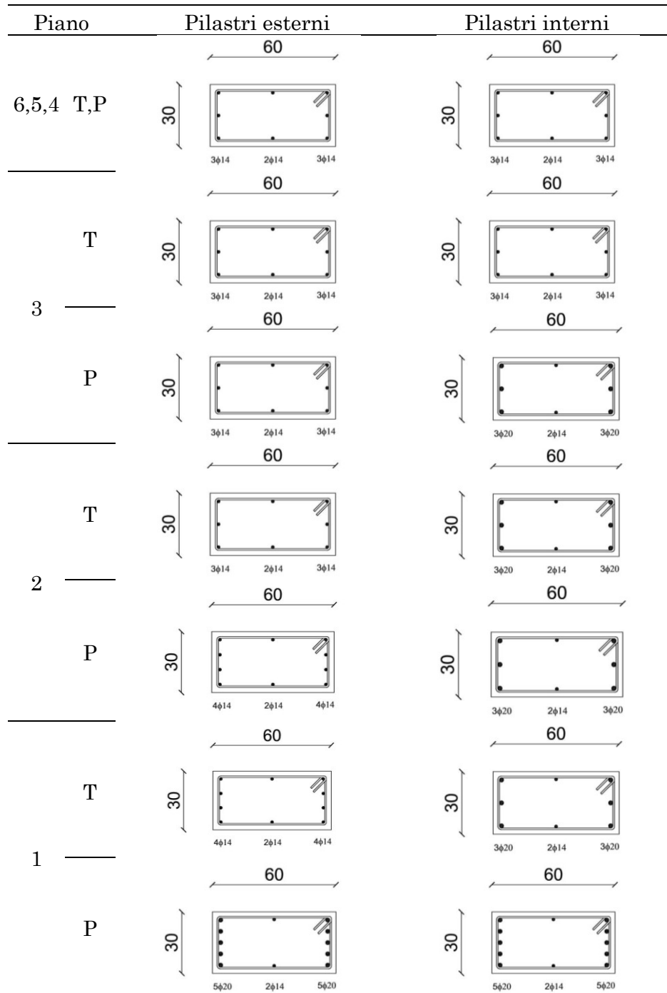
Figura 37 – Sezioni dei pilastri per il telaio progettato per bassa sismicità
