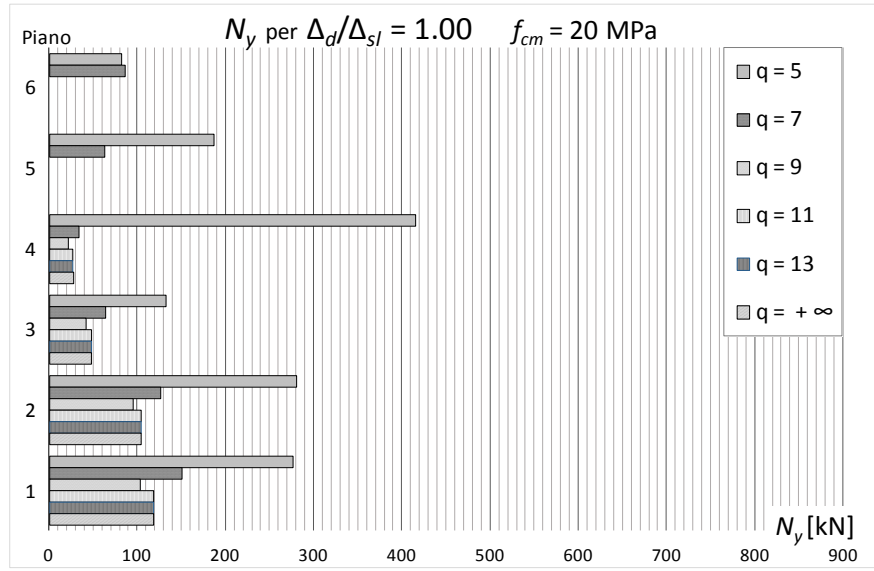
Figura 122 – Resistenza allo snervamento per progetti sul telaio AS ( f_{cm} = 20 MPa) con (\Delta_d / \Delta_{SL})_i = 1.0 al variare di q
