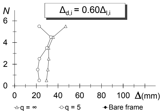
Figura 76 – Massima domanda di spostamenti di interpiano \Delta per il telaio CV2 con f_{cm} = 20 MPa adeguato, con (\Delta_d/\Delta_{SL})_i = 0.60
