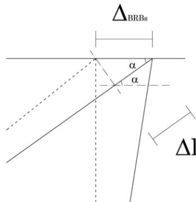
Figura 20 – Drift \Delta_{BRBs} e allungamento assiale \Delta l del BRB
