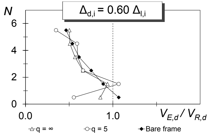
Figura 96 – Massimo rapporto V_{Ed} / V_{Rd} fra taglio sollecitante e resistente per il telaio CV1 con f_{cm} = 29 MPa adeguato, con (\Delta_d/\Delta_{SL})_i = 0.60
