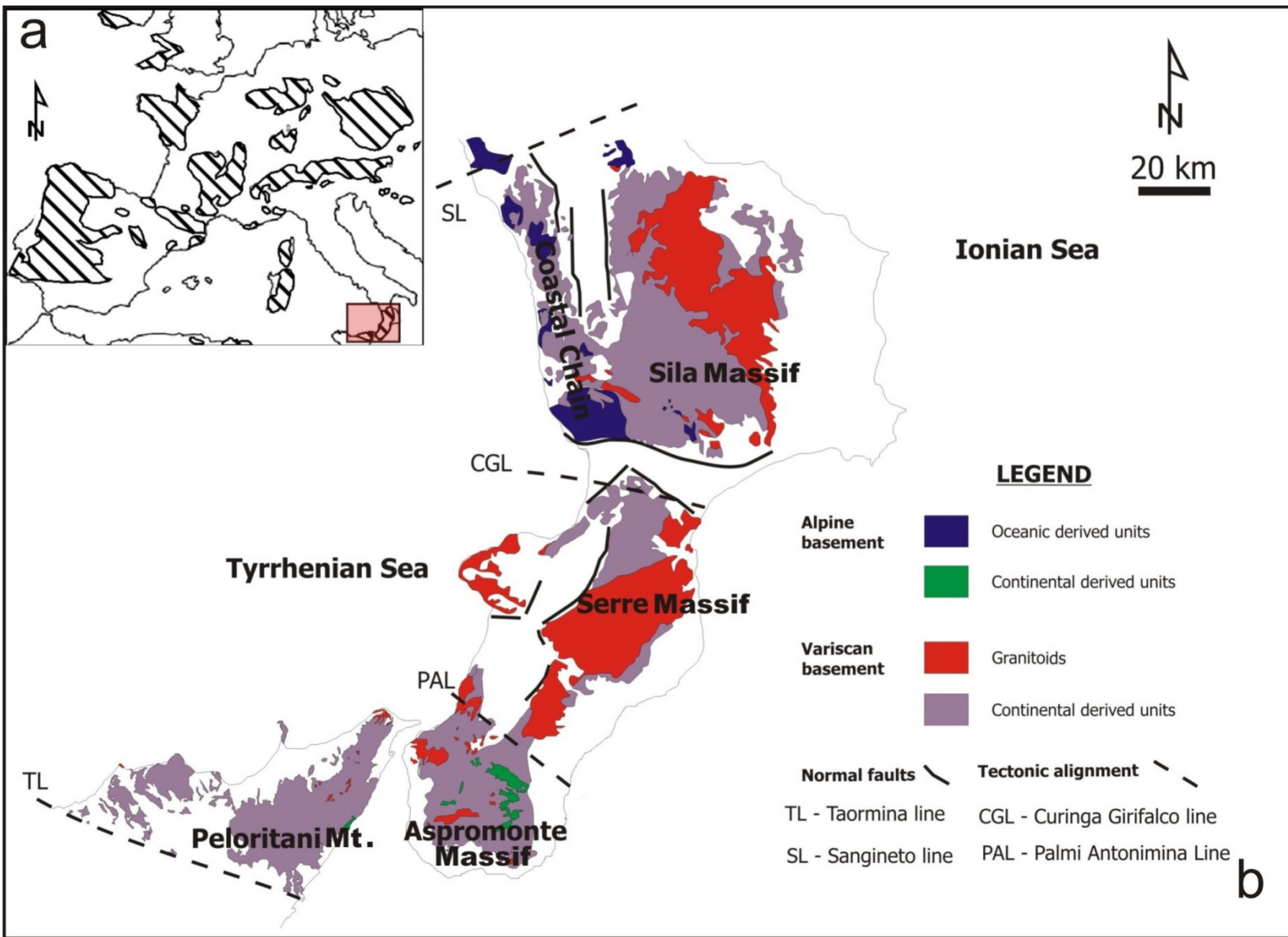
Fig.1: a) Ubicazione dei basamenti cristallini ercynici relitti nel settore occidentale del bacino mediterraneo (da von Raumer, 2002); b) Carta geologica schematica del basamento cristallino Calabro-Peloritano (da Angi et al., 2010)
