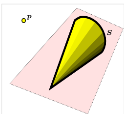
Base locus scheme \mathcal{B}(\mathcal{J}_{15}^5)
