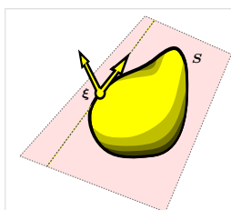
Base locus scheme \mathcal{B}(\mathcal{J}_8^5)
