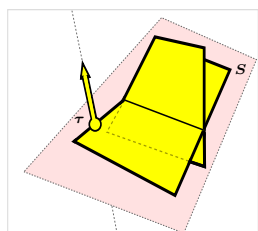
Base locus scheme \mathcal{B}(\mathcal{J}_6^5)
