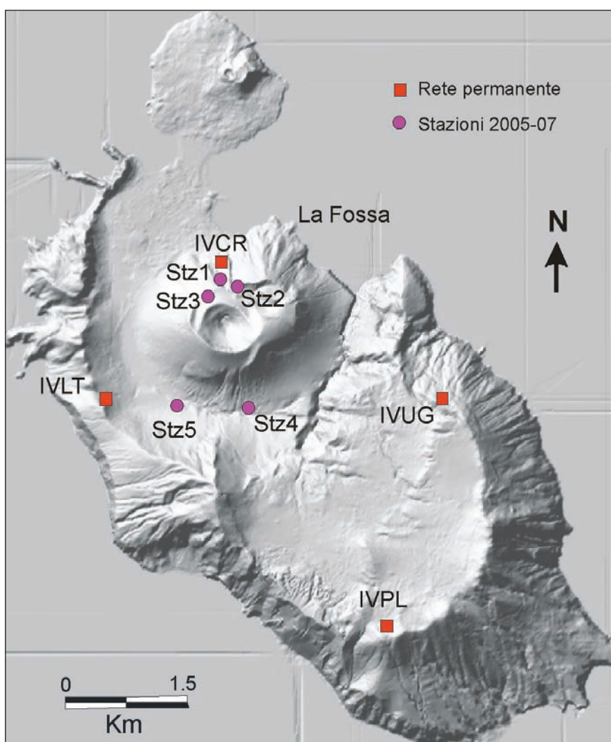
Figura 2 Mappa delle stazioni sismiche a Vulcano. I cerchi fucsia rappresentano le nuove stazioni, i quadrati rossi rappresentano le stazioni pre-esistenti.
