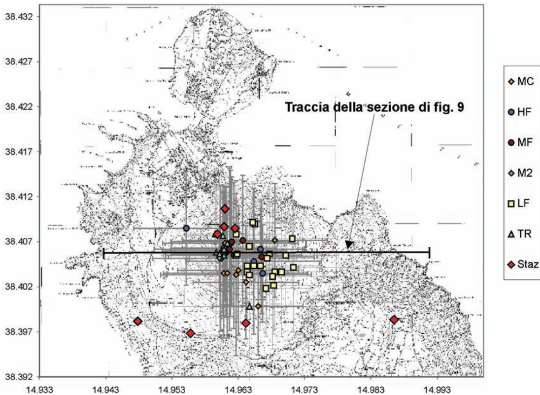
Figura 8 Mappa epicentrale e sezione E-W dei 55 eventi localizzati. Figure 8 Epicentral map and E-W cross section of the 55 located events.
