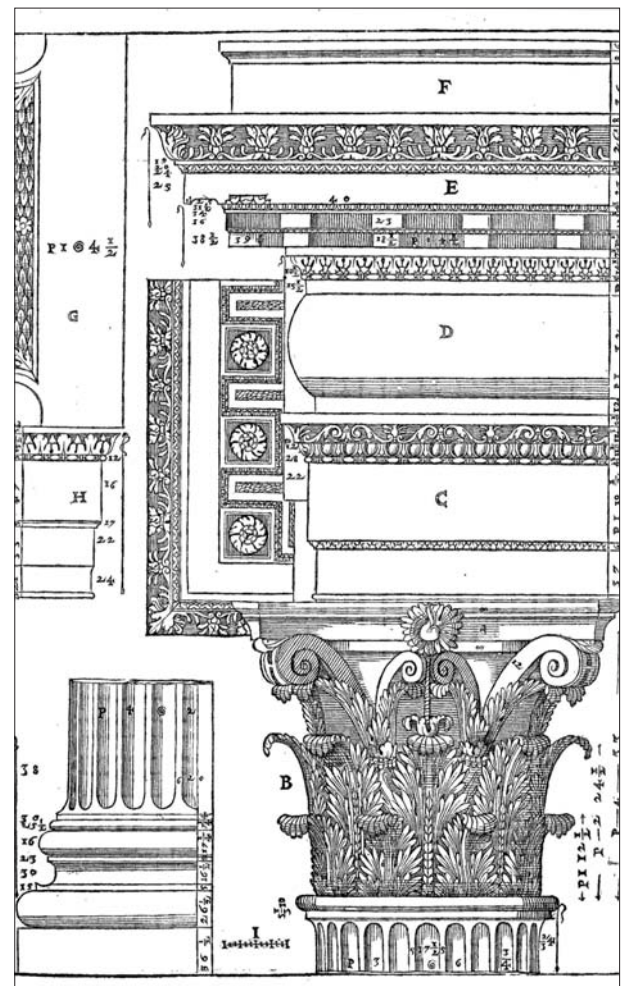
445. 446. Tempio di Giove. Tempio di Marte. Andrea Palladio., I Quattro Libri Dell'Architettura , appresso Domenico dè Franceschi, Venetia 1570, quarto libro pag. 47-60.
