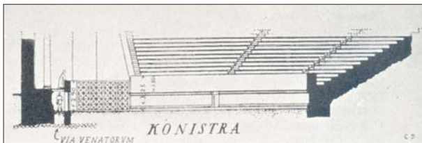
336. Stobi. Sezione del teatro nella sua seconda fase. (Saria)
