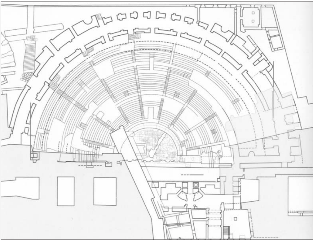
424. Pianta del teatro di Catania.
