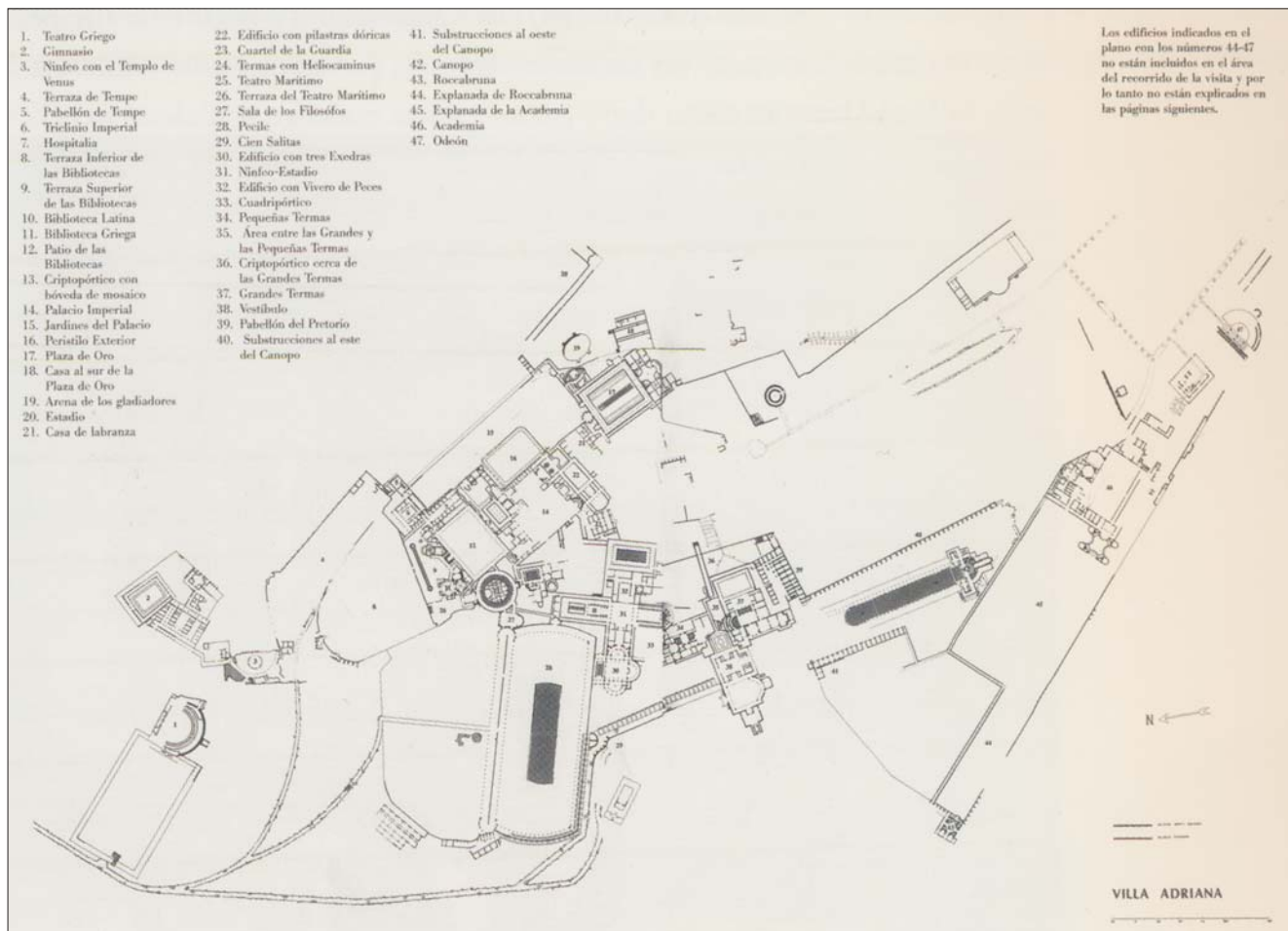
123. Tivoli. Villa Adriana, pianta con gli ambienti principali.
