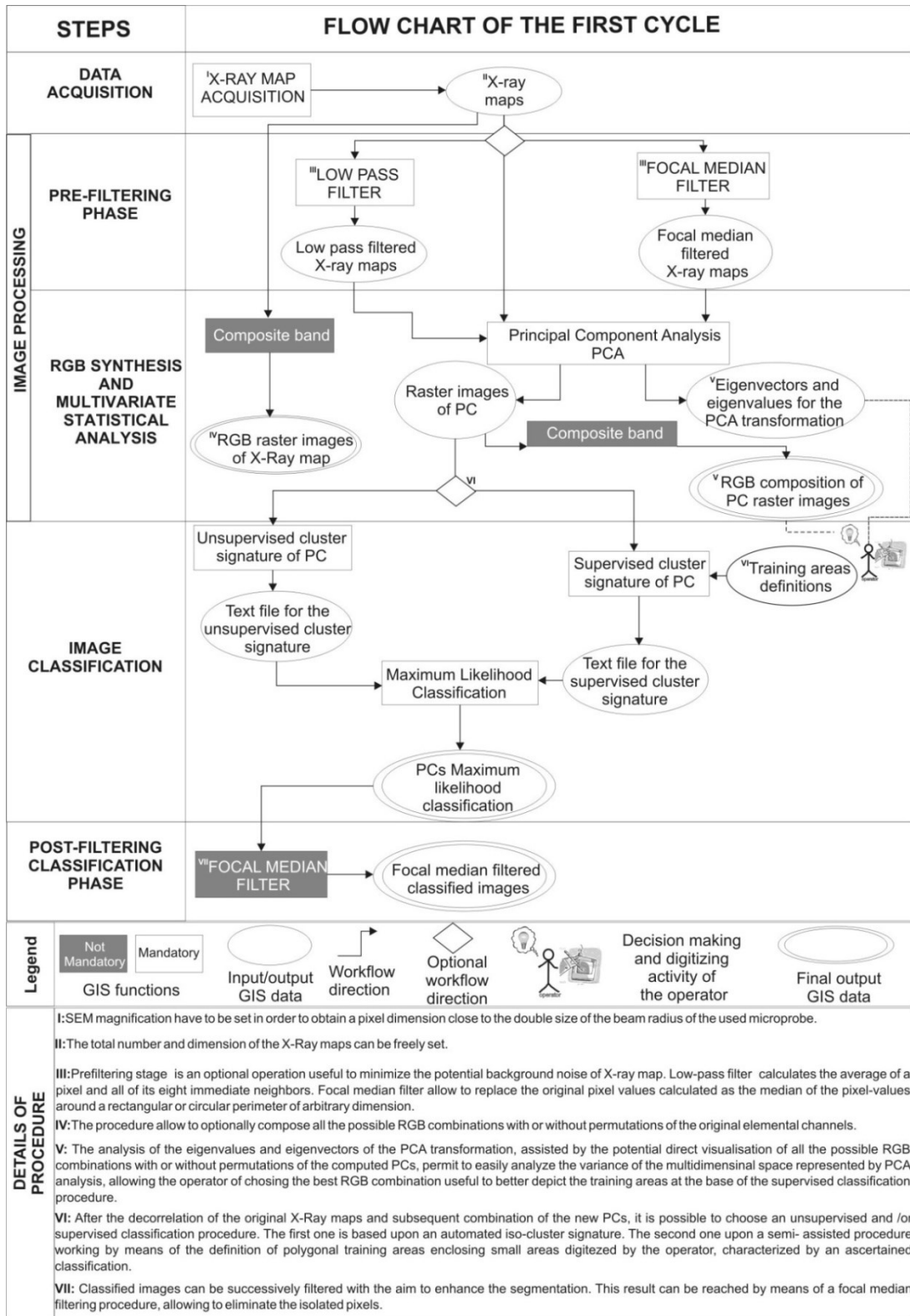
Figura 62 – Flow chart della procedura implementate nell’X-Ray Map Analyzer – (Primo Ciclo) (Ortolano et al., submitted)
