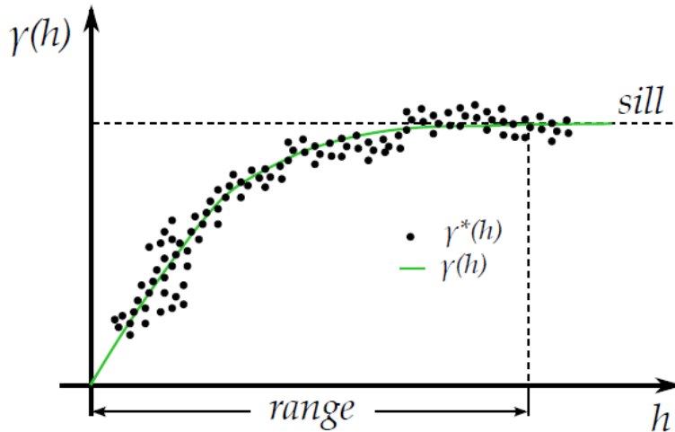
Figura 23- Variogramma sperimentale con valore di soglia fittato dal variogramma
