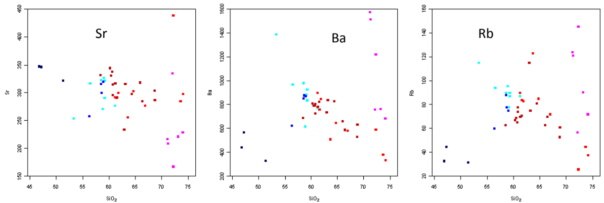
Figura 36 - Diagrammi di variazione binaria relativi a Sr, Ba e Rb.
