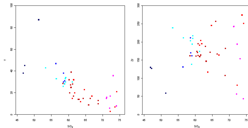
Figura 37 - Diagrammi di variazione binaria relativi a Y e Zr
