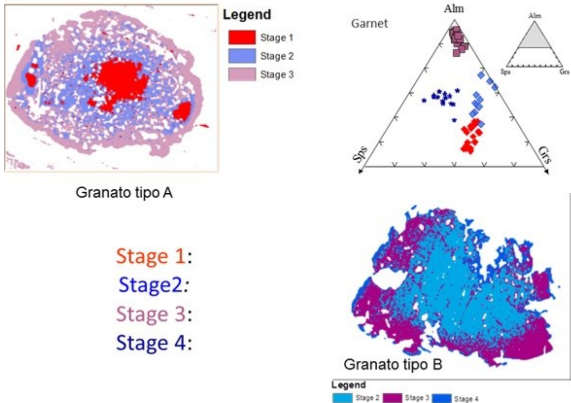
Figura 72 - Classificazione della zoneografia mineralogica nei granati di tipo "A" e di tipo "B"
