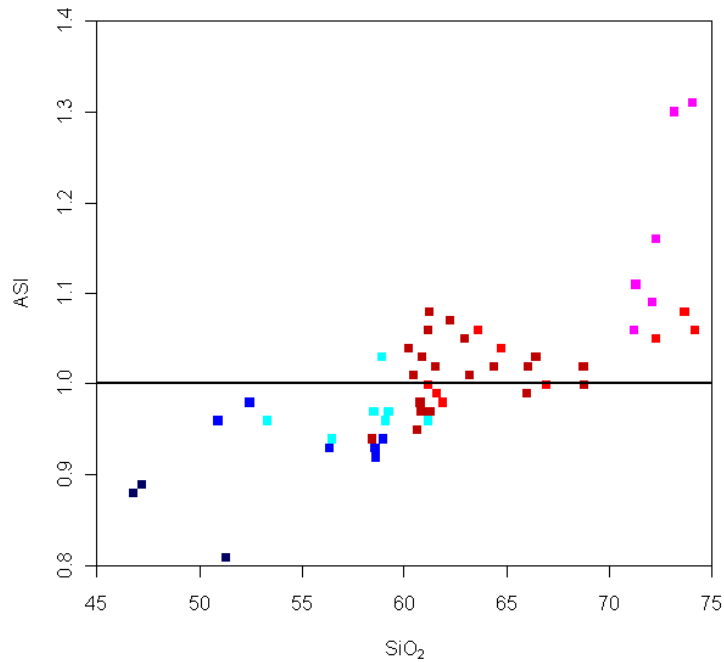
Figura 33 - Diagramma SiO 2 vs. ASI
