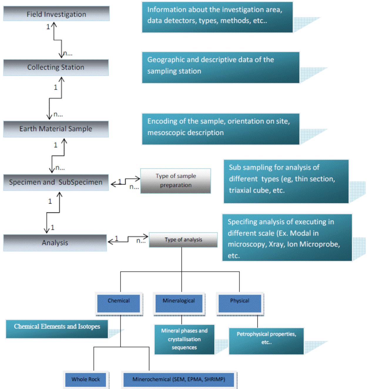
Figura 20 - FOS2MAN – Schema semplificato del modello Entità - Relazione
