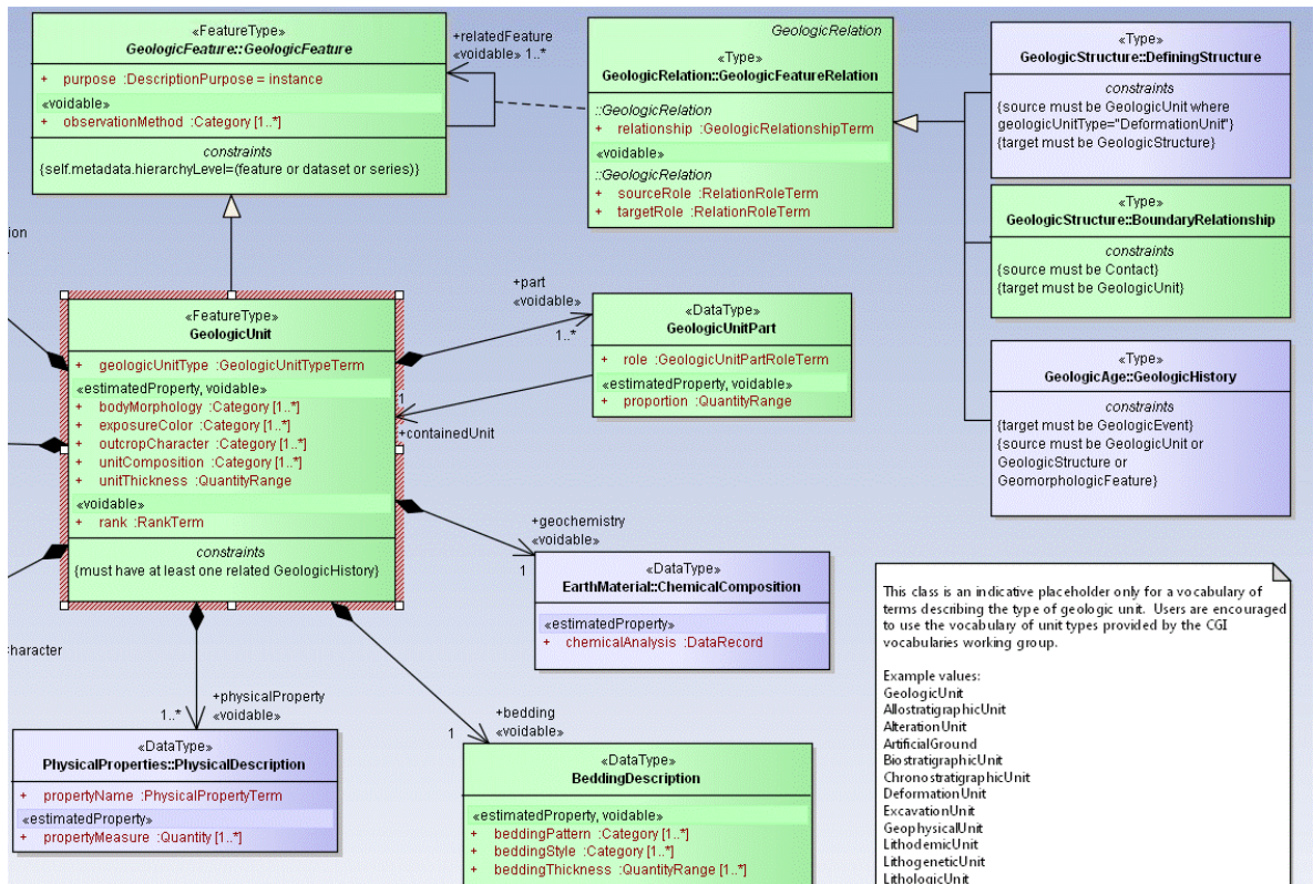
Figura 12 – Schema relazionale GeoSciML v. 3.2 – Geologic Unit (per il significato dei simbolismi vedi nota 1)
