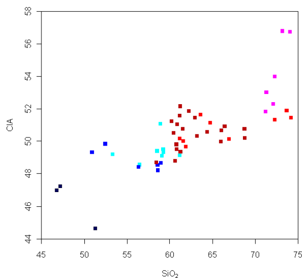
Figura 38 - Diagramma di variazione binaria relativo al CIA.
