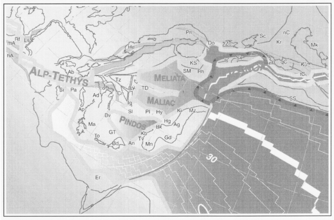
Figura 1- Ricostruzione del Giurassico medio (Aaleniano, 180 Ma). I bacini oceanici Pindos, Maliac e Meliata rappresentano back-arc basins formati in seguito alla chiusura della Paleotetide e al roll-back dello slab che subduce sotto il margine Europeo. Legenda: Ab, Alboran; Ad, Adria s. s.; Ag, Aladag; An, Antalya; Ap, Apulia s. s.; Bd, Beydaghlari; Bk, Bolkardag; By, Beyshehir; Bv, Budva; Cn, Carnic-Julian; Do, Dobrogea; eP, east Pontides; Er, Eratosthen; gC, great Caucasus; Gd, Geydag; GT, Gavrovo-Tripolitza; hA, high-Atlas; He, Helvetic rim basin; Hg, Huglu; Hy, Hidra; Ig, Igal trough; Is, Instabul; Jv, Juvavic; Kb, Karaburun; Ki, Kirshehir; Ko, Korab; KS, Kotel-Stranja; Ku, Kura; Lo, Lombardian; Ls, Lusitanian; mA, middle Atlas; Ma, Mani; Mk, Mangyshlak rift; Mn, Menderes; Mz, Munzur dag; nC, north Caspian; Pa, Panormides; PI, Pelagonian; Pn, Pienniny rift; Rf, Rif external; Rh, Rhodope; Si, Sicani; Sl, Slavonia; Sc, Scythian platform; Sk, Sakarya; SM, Serbo-Macedonian; SS, Sanandaj-Sirjan; Tc, Transcaucasus; TD, Trans-Danubian; To, Talea Ori; Tv, Tavas+Tavas seamount; Tz, Tizia (da Stampfli et al., 2002).
