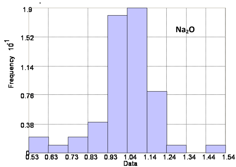
Figura 47 - Frequenza di distribuzione del Na 2 O
