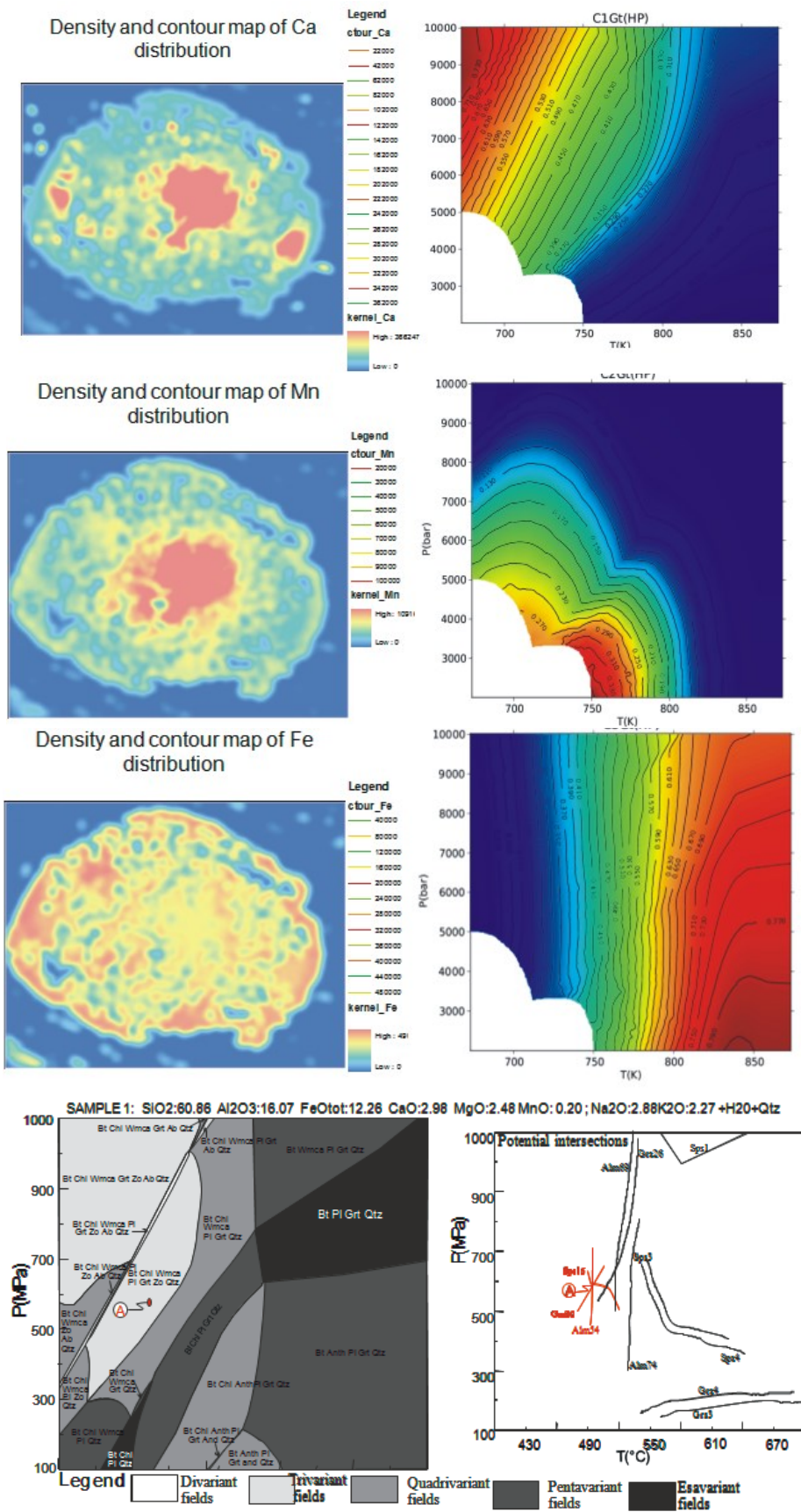
Figura 73 – Distribuzione zoneografica del granato di tipo A e seguenti vincoli termobarici
