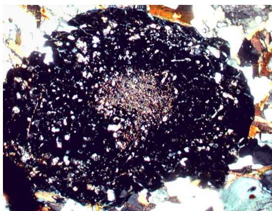
Figura 65 - Osservazioni al microscopio ottico dei 2 campioni di granato appartenenti ai micascisti granatiferi del Complesso di Mammola: A) Granato con zonatura di tipo progradata Nicols X; B) Granato con strutture di tipo retrogrado Nicols //
