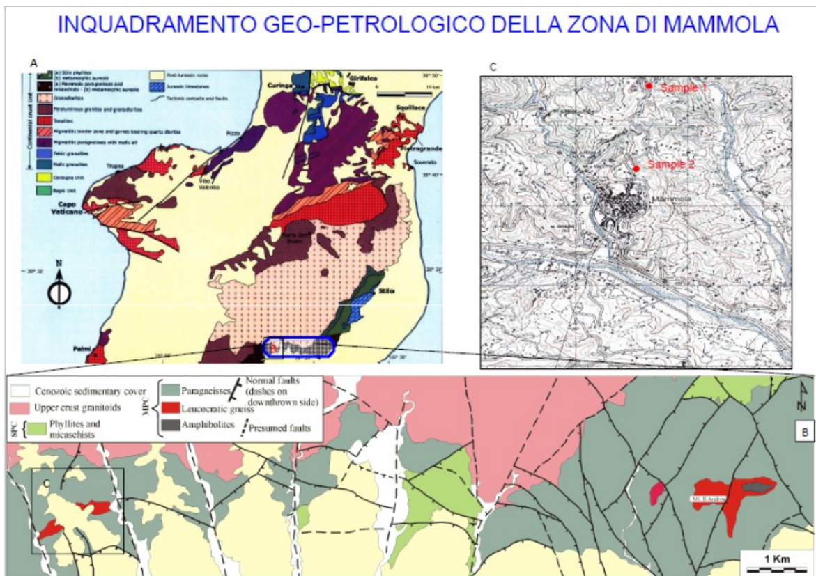
Figura 55- Inquadramento geo-petrologico dell'area studio: A) Carta geologica schematica del Massiccio delle Serre (Caggianelli et al., 2013); B) Carta Geologica schematica della zona di Mammola (Angi et al., 2010); C) Localizzazione dei punti di campionamento dei micascisti granatiferi analizzati
