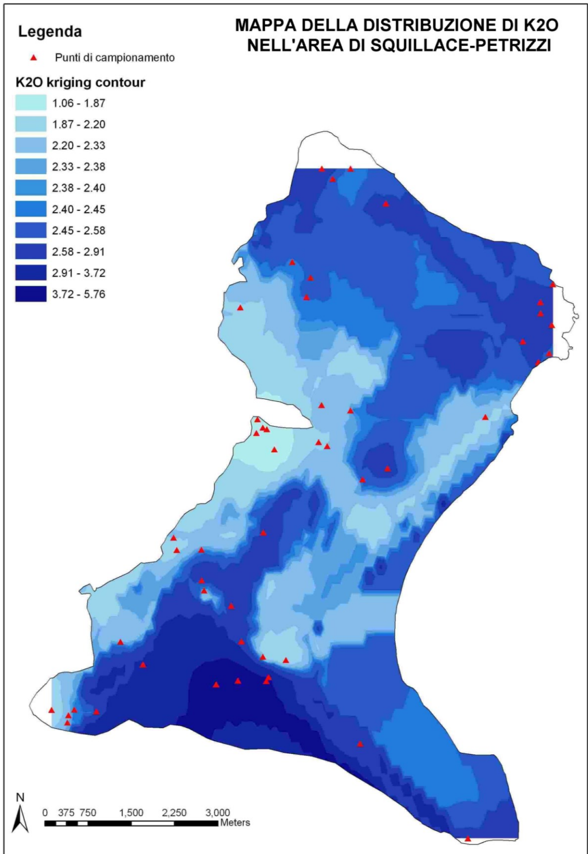
Figura 46 - Kriging Ordinario del K2O
