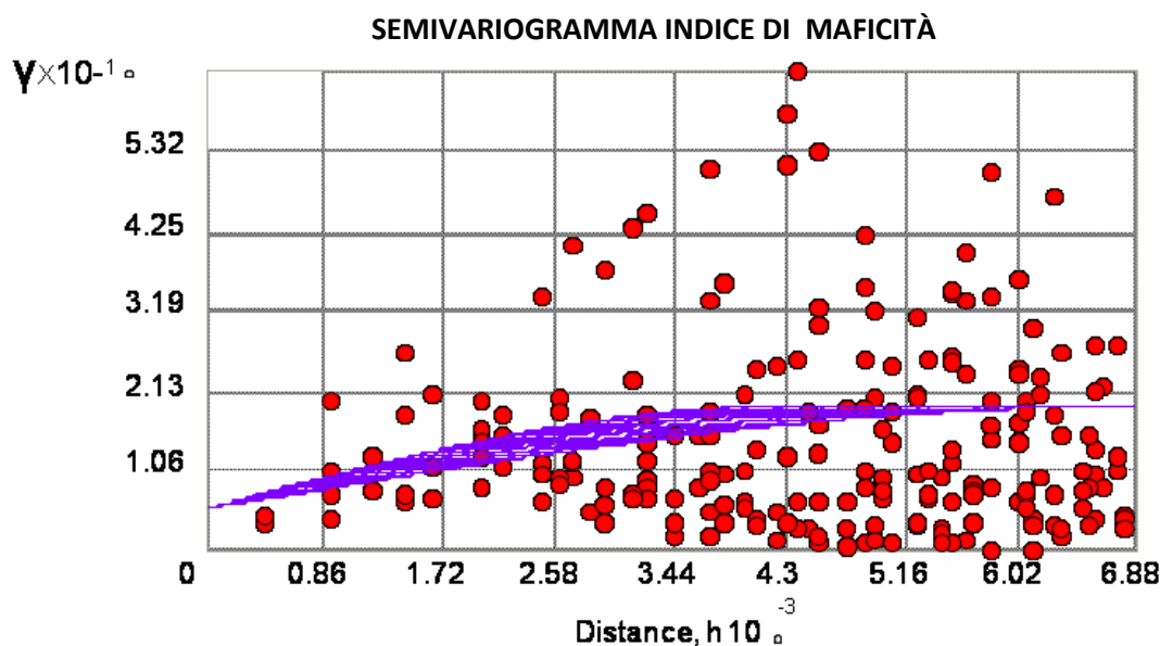
Figura 51 - Semivariogramma dell'Indice di Maficità
