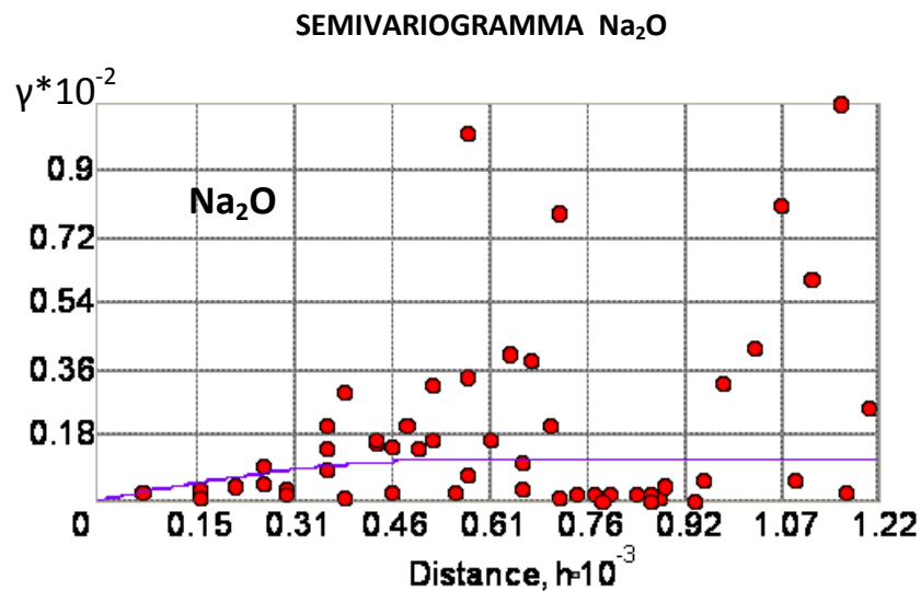
Figura 49 - Semivariogramma del Na 2 O
