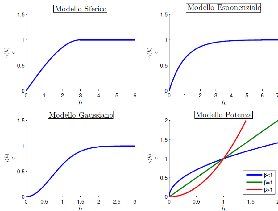
Figura 24 - Grafici qualitativi dei variogrammi teorici elementari più utilizzati in geostatistica
