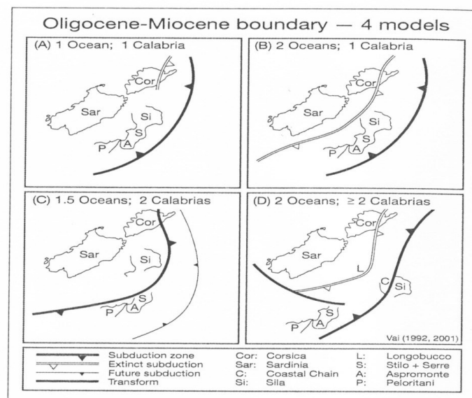
Figura 4 - Schema delle possibili configurazioni dei margini di placca durante il Terziario medio-superiore nelle ipotesi in cui la Calabria sia costituita da uno o due terreni, e limitata da uno o due oceani. In (C), "1,5 oceans" significa un unico oceano nella zona della Sila e due oceani nella zona Stilo-Serre-Aspromonte-Peloritani (da Alvarez & Shimabukuro, 2009).
