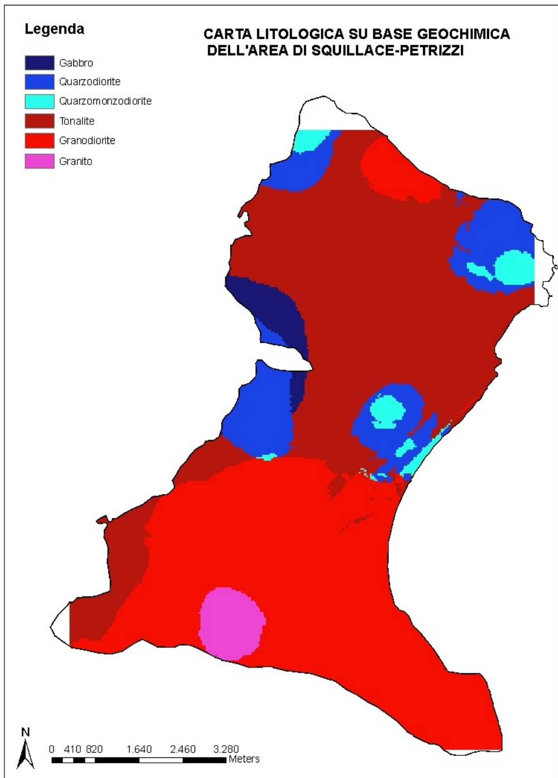
Figura 53 - Mappa litologica ricostruita mediante l'algoritmo di classificazione basato su TAS Middlemost 1985
