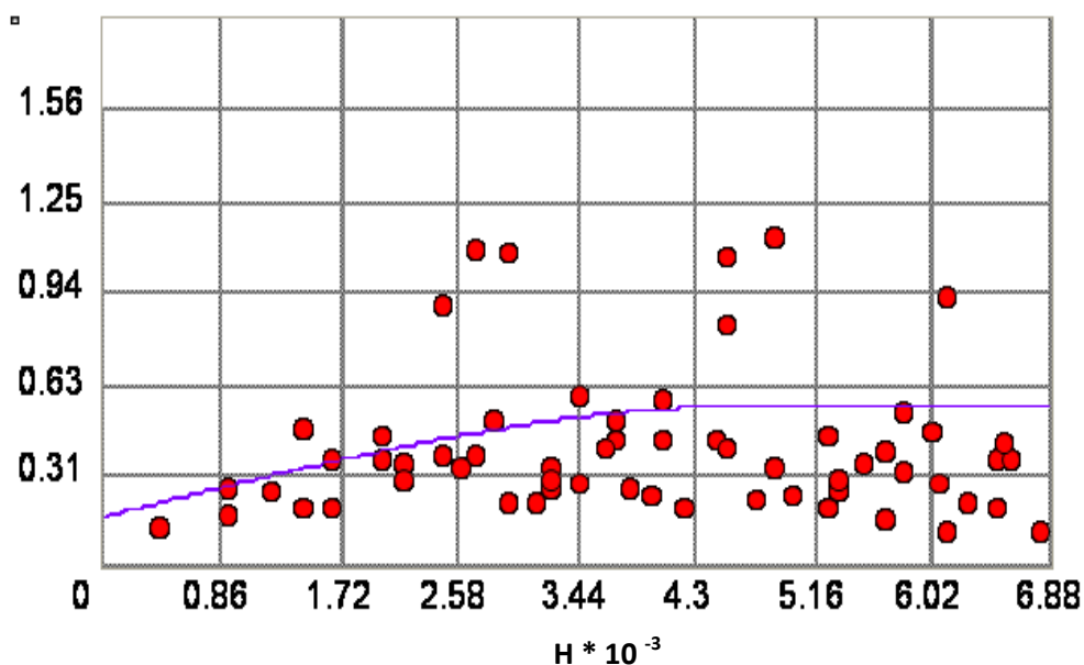
Figura 41 - Semivariogramma relativo alla \text{SiO}_2
