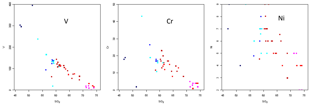
Figura 35 - Diagrammi di variazione binaria relativi a V, Cr e Ni
