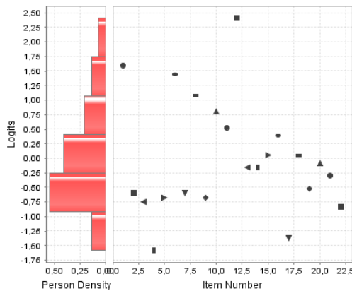
Fig. 2 Mappa degli item del LIEP test.
