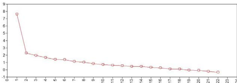
Fig. 1 Scree-plot degli autovalori del LIEP Test.
